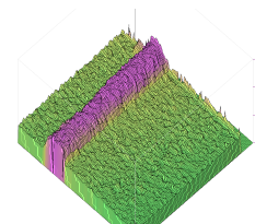
3D-Bild einer Schweißnahtvermessung
